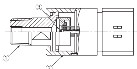
内部構造図 INTERNAL STRUCTURE PA-750 (R 1/4)
