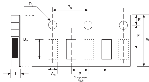
0201/0402 CASE SIZE
