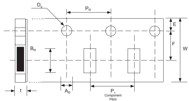
0603/0805 CASE SIZE
