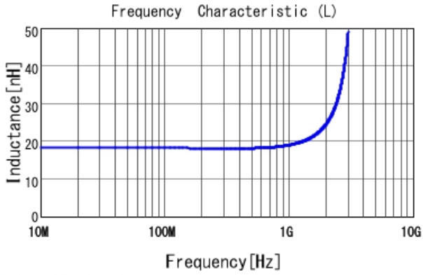
■ LQP15MN18NG02 L
