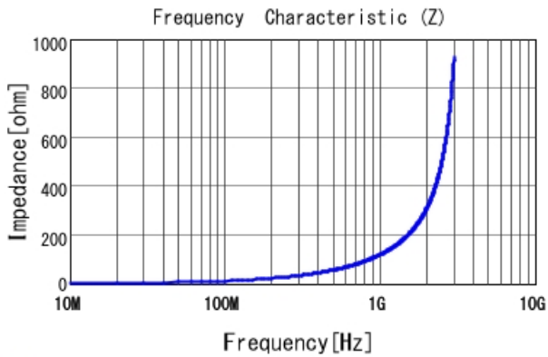
■ LQP15MN18NG02 |Z|
