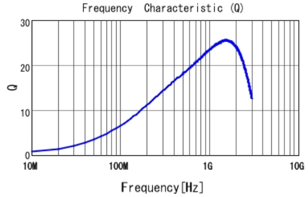
■ LQP15MN18NG02 Q
