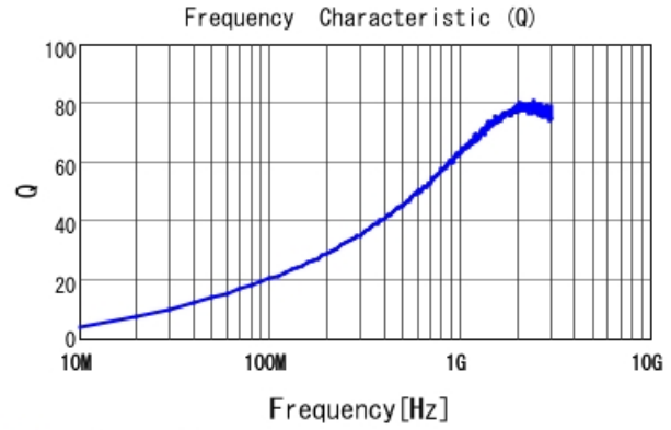
■ LQW15AN24NJ00 Q
