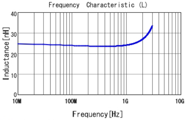
■ LQW15AN24NJ00 L
