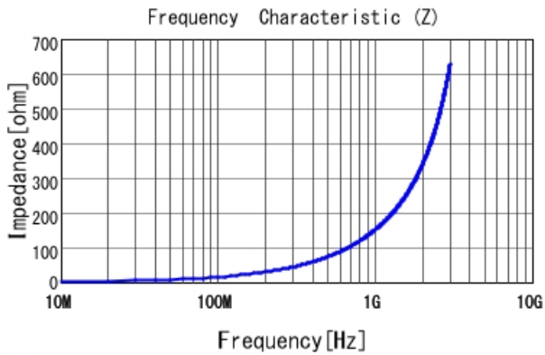
■ LQW15AN24NJ00 |Z|
