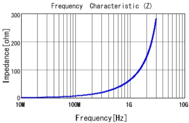
■ LQP03TN10NH02 |Z|
