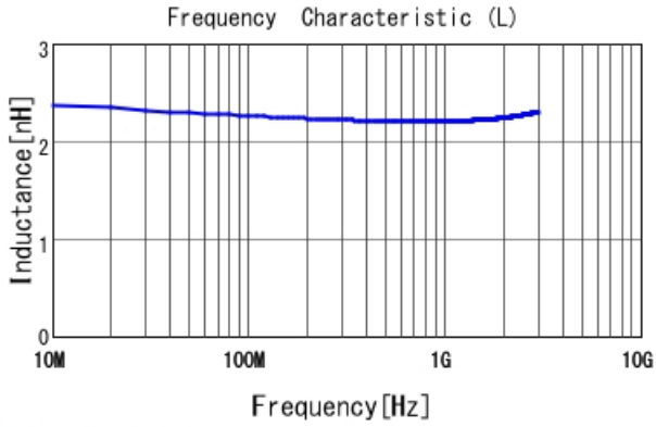
■ LQW15AN2N4B00 L
