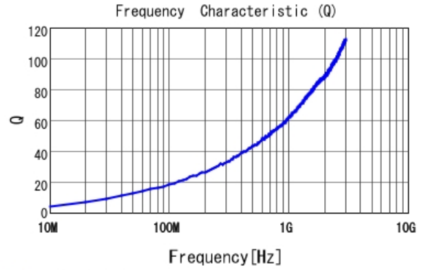
■ LQW15AN2N4B00 Q
