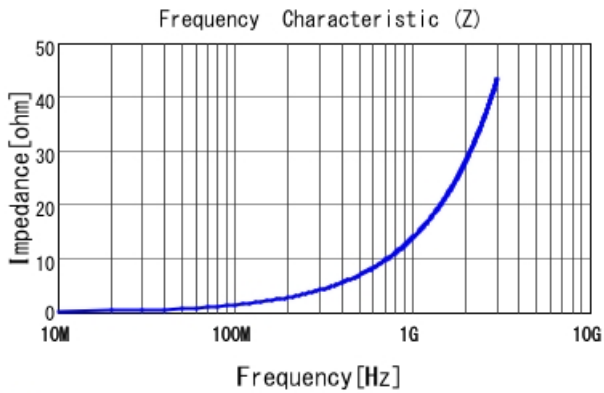
■ LQW15AN2N4B00 |Z|
