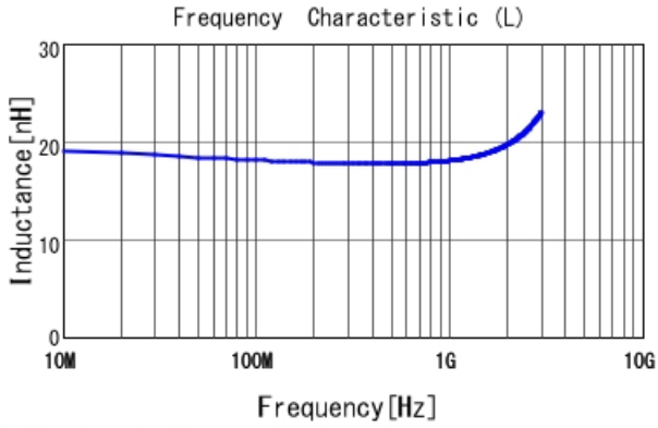
■ LQW15AN18NJ00 L
