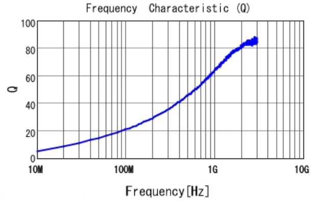
■ LQW15AN18NJ00 Q
