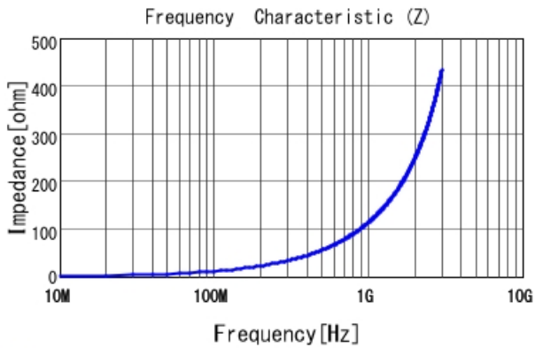
■ LQW15AN18NJ00 |Z|
