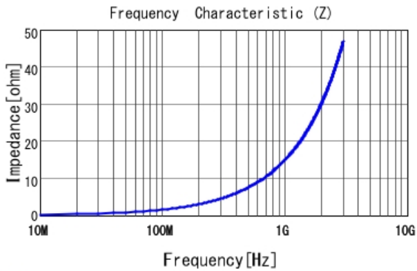
■ LQW15AN2N5B00 |Z|
