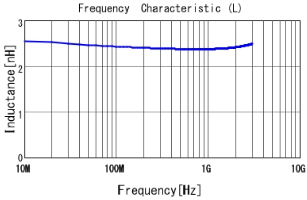
■ LQW15AN2N5B00 L
