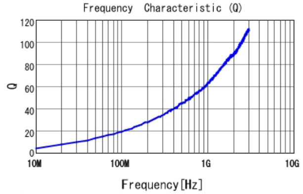
■ LQW15AN2N5B00 Q
