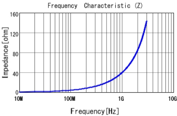
■ LQP15MN6N2B02 |Z|
