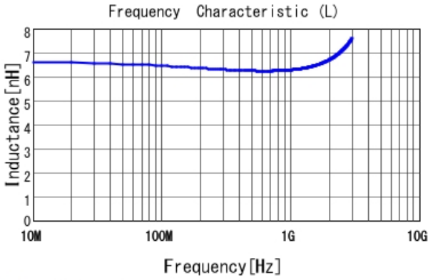
■ LQP15MN6N2B02 L
