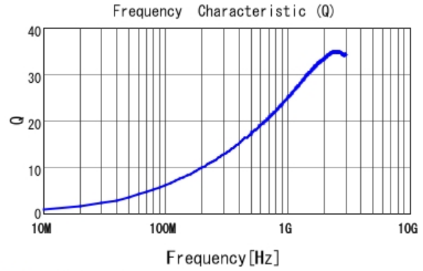
■ LQP15MN6N2B02 Q
