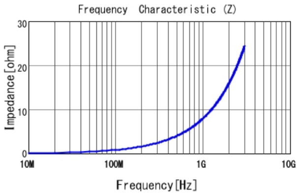
■ LQW15AN1N3C10 |Z|
