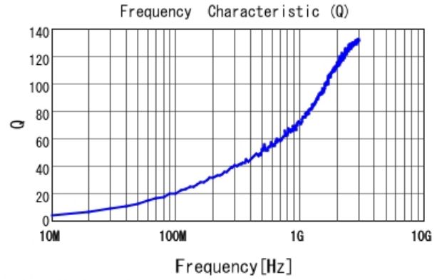
■ LQW15AN1N3C10 Q
