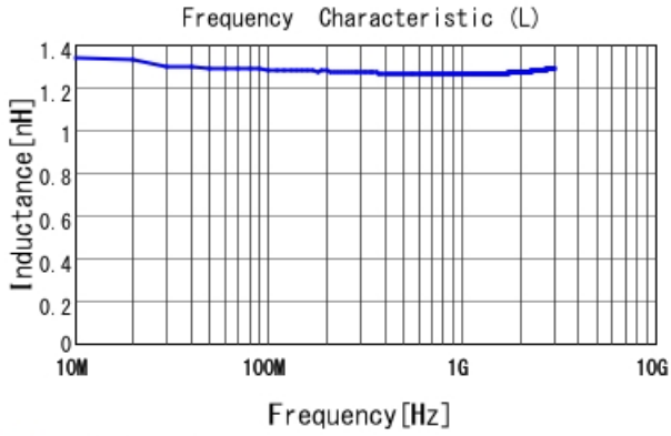
■ LQW15AN1N3C10 L
