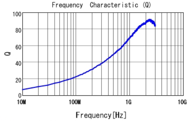
■ LQW15AN12NJ00 Q
