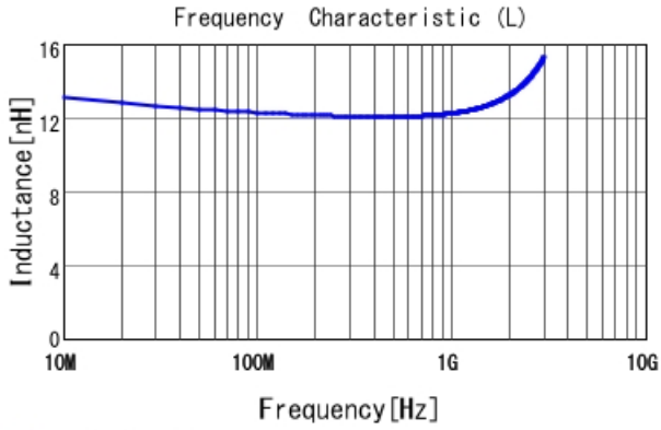
■ LQW15AN12NJ00 L
