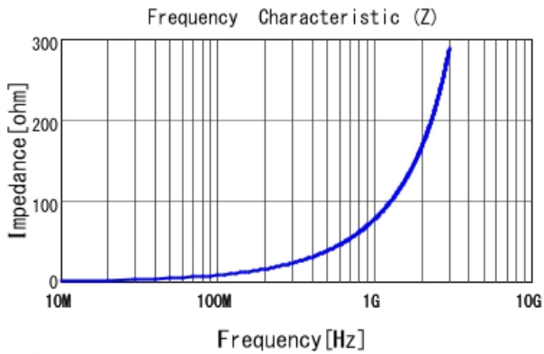
■ LQW15AN12NJ00 |Z|
