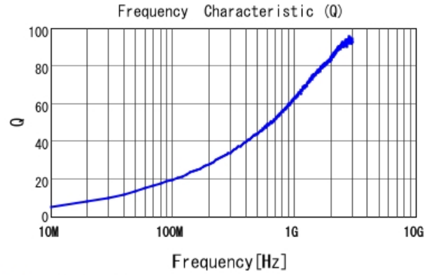
■ LQW15AN11NJ00 Q
