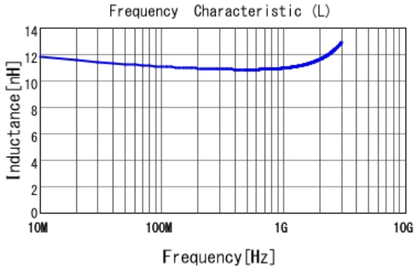
■ LQW15AN11NJ00 L
