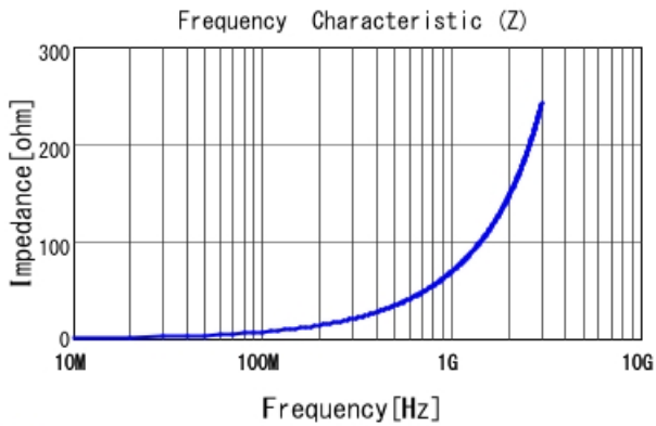
■ LQW15AN11NJ00 |Z|
