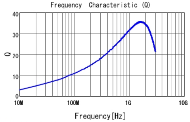
■ LQG15HN10NJ02 Q
