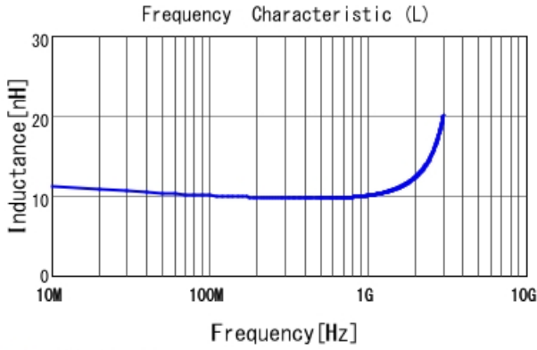
■ LQG15HN10NJ02 L
