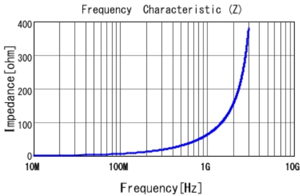
■ LQG15HN10NJ02 |Z|
