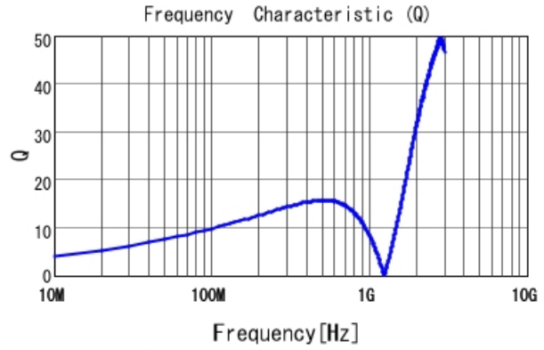
■ LQG15HN68NJ02 Q
