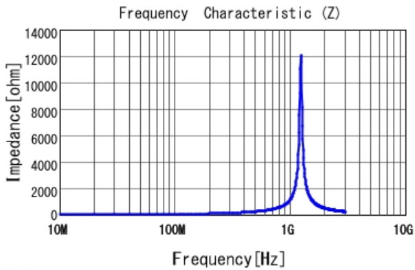
■ LQG15HN68NJ02 |Z|
