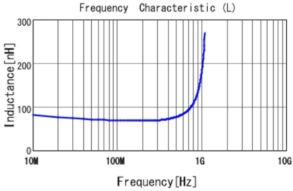
■ LQG15HN68NJ02 L
