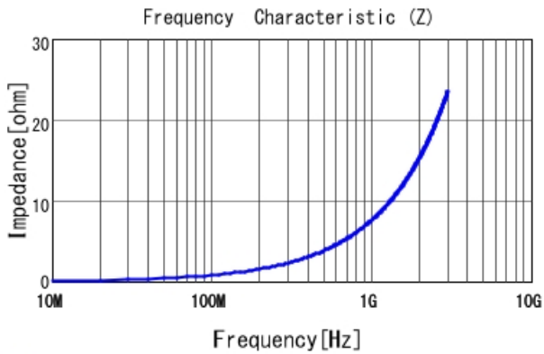
■ LQG15HN1N2S02 |Z|
