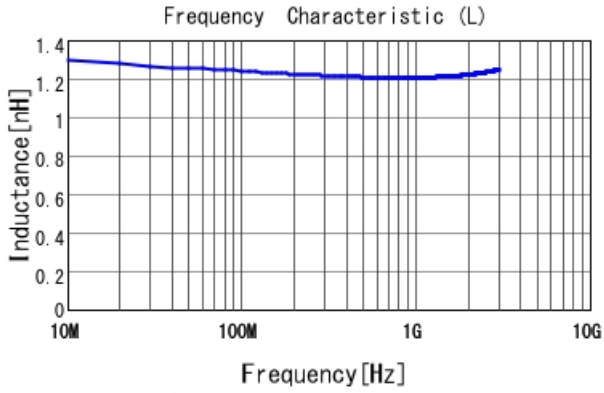
■ LQG15HN1N2S02 L
