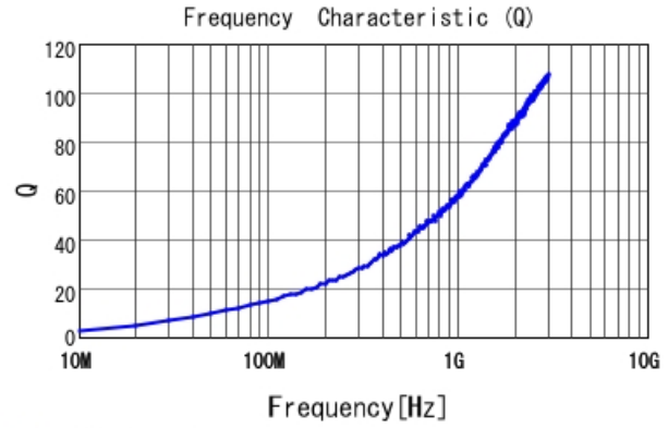
■ LQG15HN1N2S02 Q
