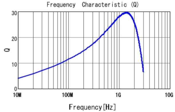
■ LQG15HS12NJ02 Q
