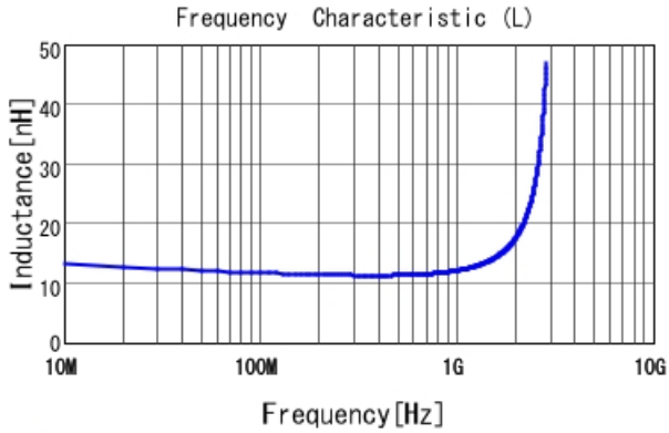
■ LQG15HS12NJ02 L
