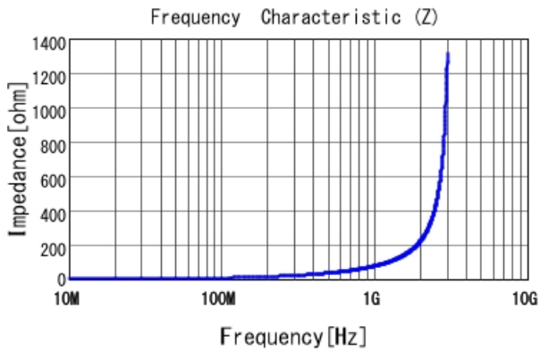
■ LQG15HS12NJ02 |Z|
