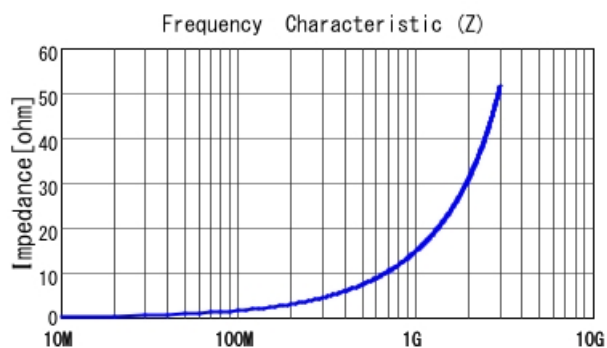
■ LQG15HN2N4S02 |Z|
