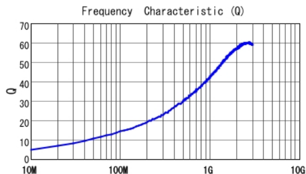
■ LQG15HN2N4S02 Q
