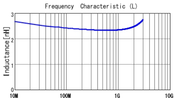
■ LQG15HN2N4S02 L
