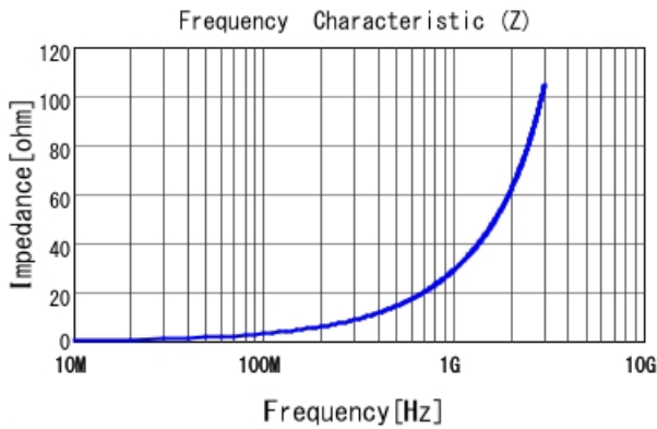
■ LQG15HN4N7S02 |Z|
