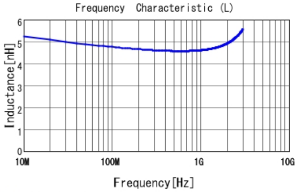
■ LQG15HN4N7S02 L
