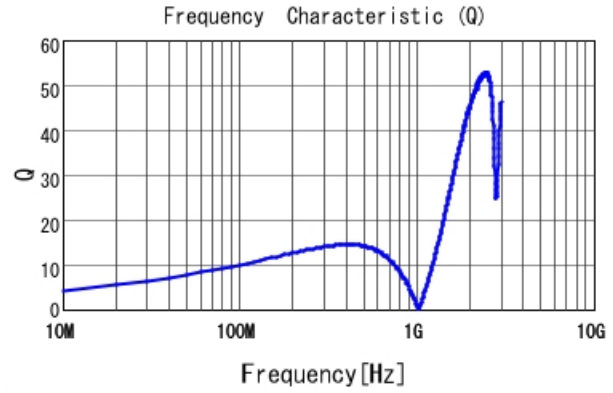
■ LQG15HN82NJ02 Q
