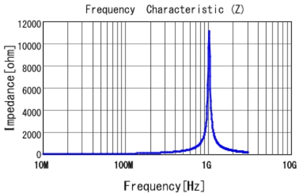
■ LQG15HN82NJ02 |Z|
