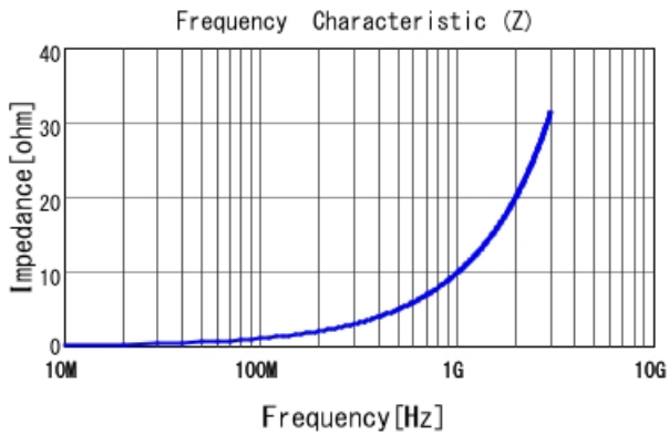
■ LQG15HN1N6S02 |Z|
