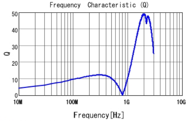
■ LQG15HNR12J02 Q
