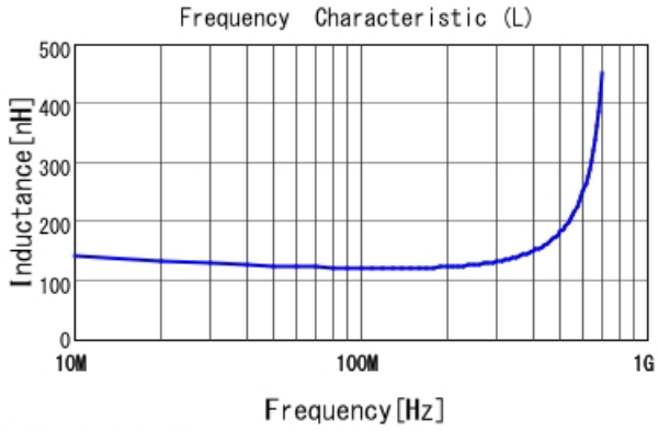
■ LQG15HNR12J02 L
