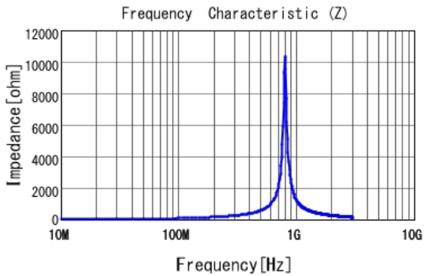
■ LQG15HNR12J02 |Z|
