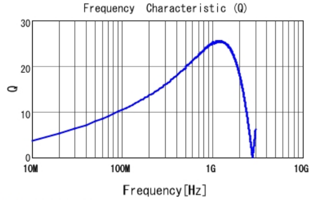
■ LQG15HS18NJ02 Q
