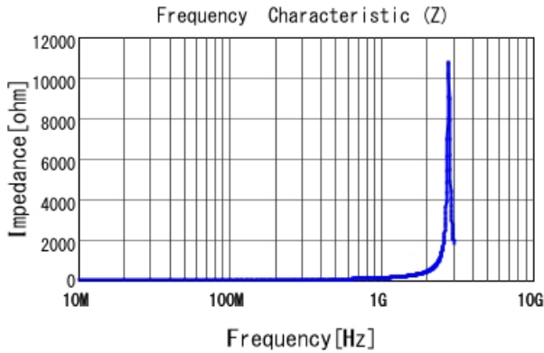
■ LQG15HS18NJ02 |Z|
