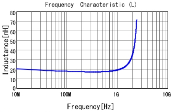
■ LQG15HS18NJ02 L
