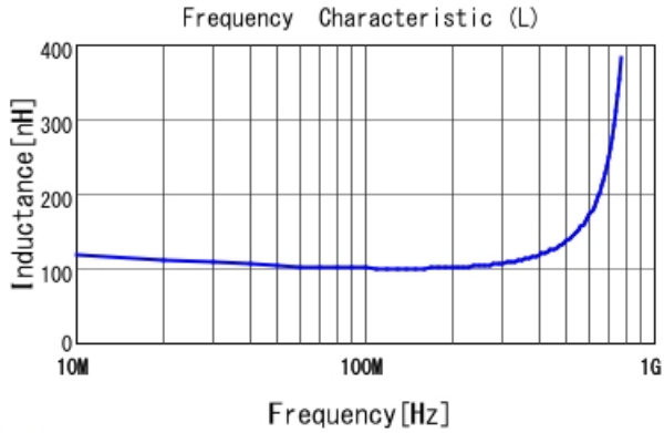
■ LQG15HNR10J02 L
