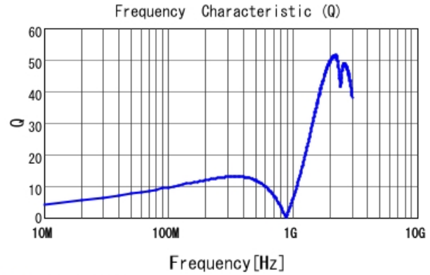
■ LQG15HNR10J02 Q
