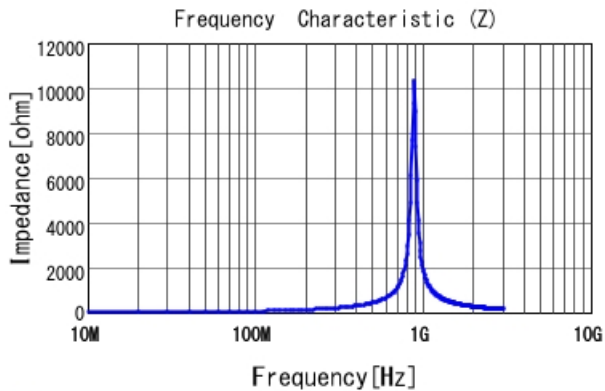
■ LQG15HNR10J02 |Z|
