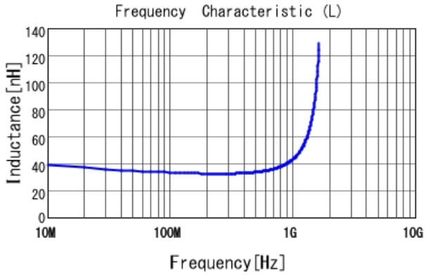
■ LQG15HN33NJ02 L
