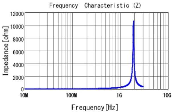
■ LQG15HN33NJ02 |Z|
