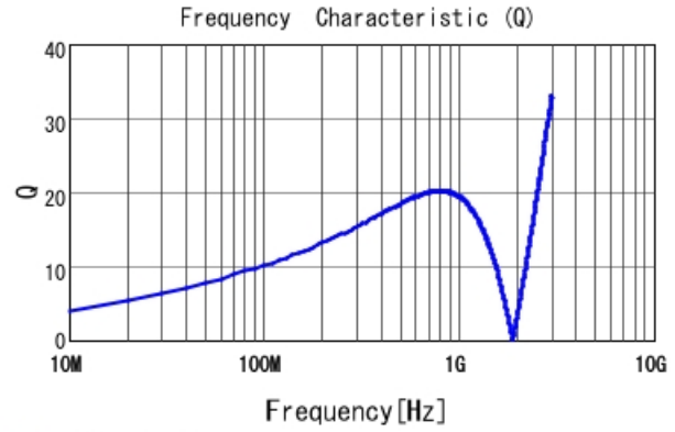
■ LQG15HN33NJ02 Q
