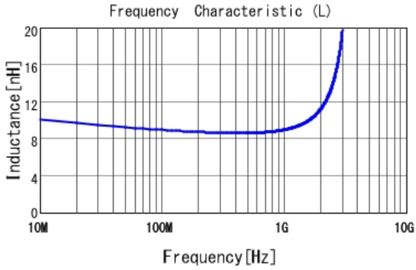
■ LQG15HN9N1J02 L
