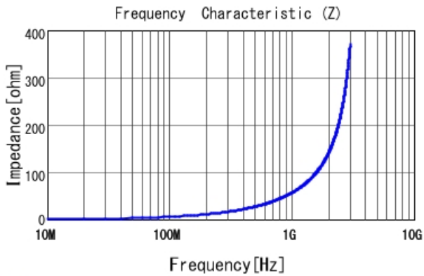
■ LQG15HN9N1J02 |Z|
