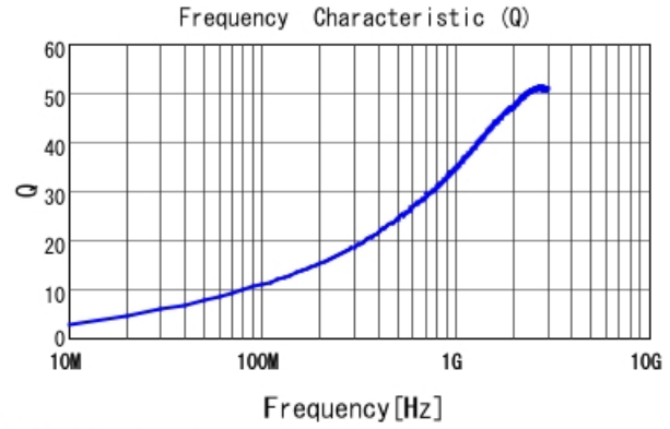
■ LQG15HN4N3S02 Q
