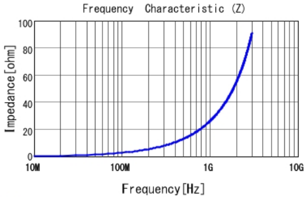
■ LQG15HN4N3S02 |Z|
