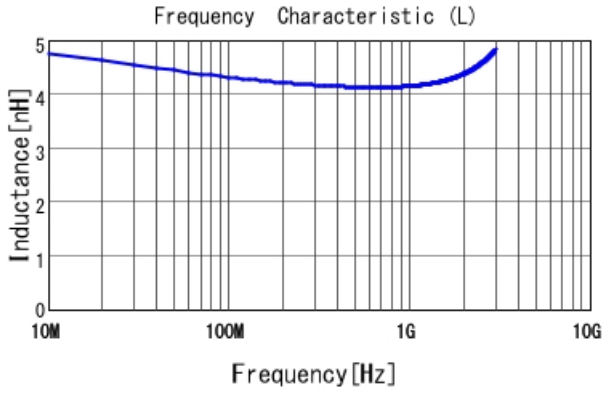
■ LQG15HN4N3S02 L
