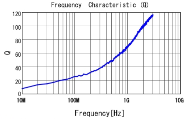
■ LQG15HN1N3S02 Q
