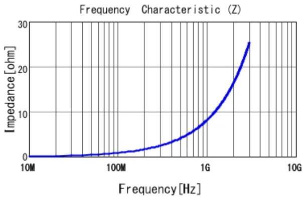
■ LQG15HN1N3S02 |Z|
