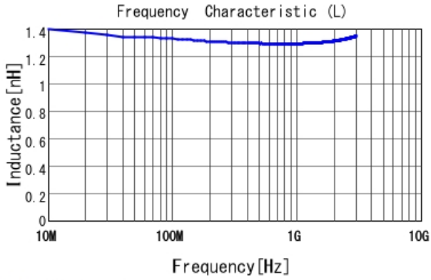
■ LQG15HN1N3S02 L
