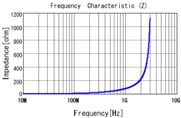
■ LQG15HN12NJ02 |Z|
