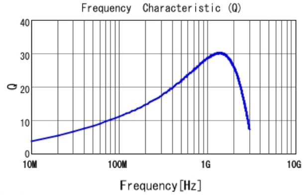
■ LQG15HN12NJ02 Q
