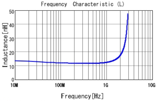
■ LQG15HN12NJ02 L
