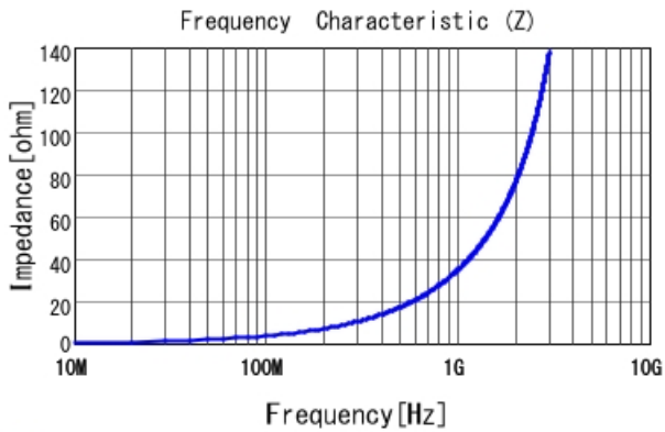
■ LQG15HN5N6S02 |Z|
