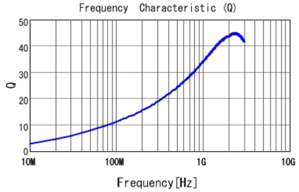
■ LQG15HN5N6S02 Q
