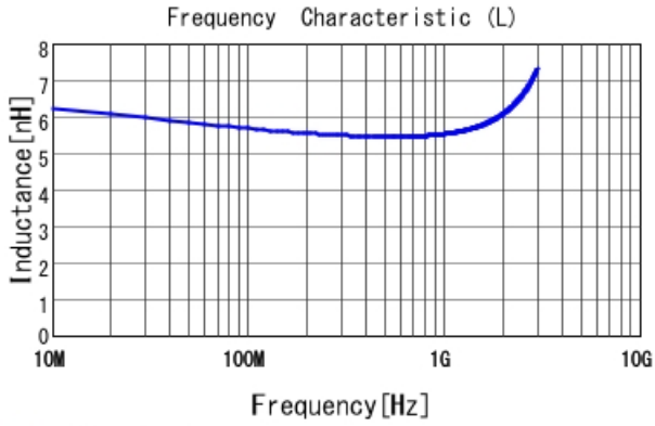
■ LQG15HN5N6S02 L
