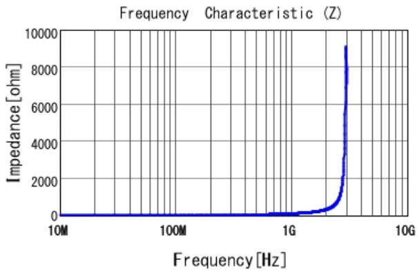
■ LQG15HN15NJ02 |Z|
