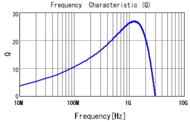
■ LQG15HN15NJ02 Q
