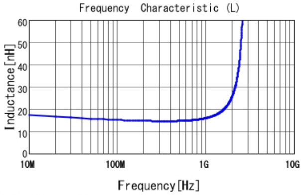
■ LQG15HN15NJ02 L
