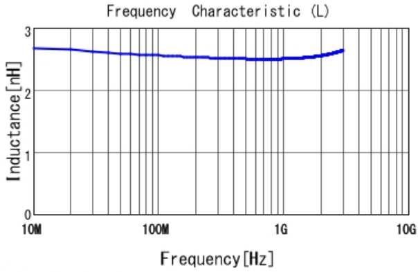
■ LQW15AN2N7B00 L
