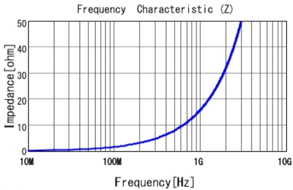
■ LQW15AN2N7B00 |Z|
