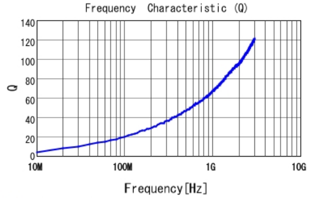
■ LQW15AN2N7B00 Q
