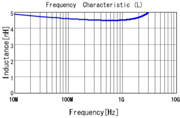
■ LQW15AN4N7B00 L
