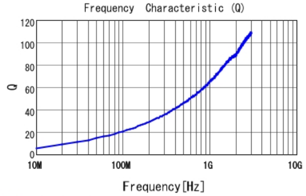
■ LQW15AN4N7B00 Q
