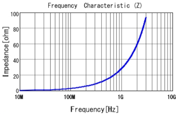
■ LQW15AN4N7B00 |Z|
