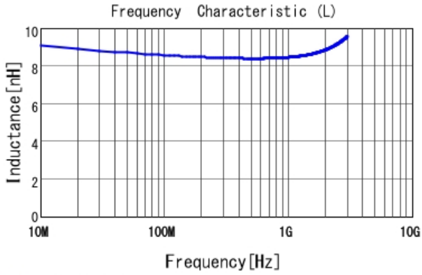
■ LQW15AN8N7G00 L
