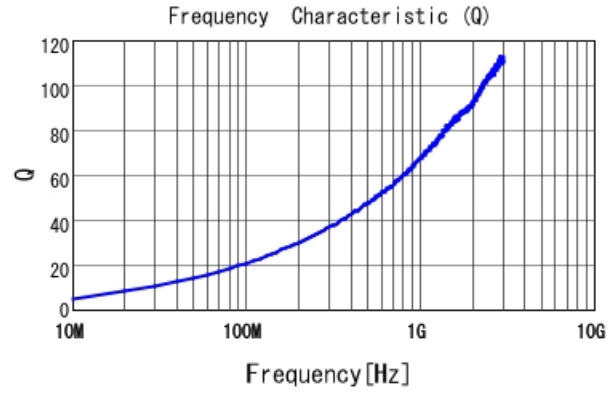
■ LQW15AN8N7G00 Q
