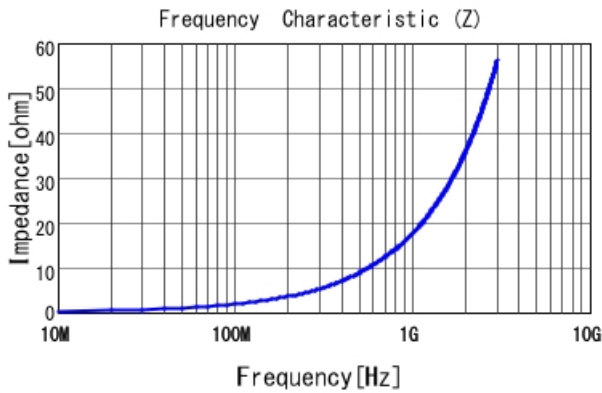
■ LQW15AN2N9B00 |Z|
