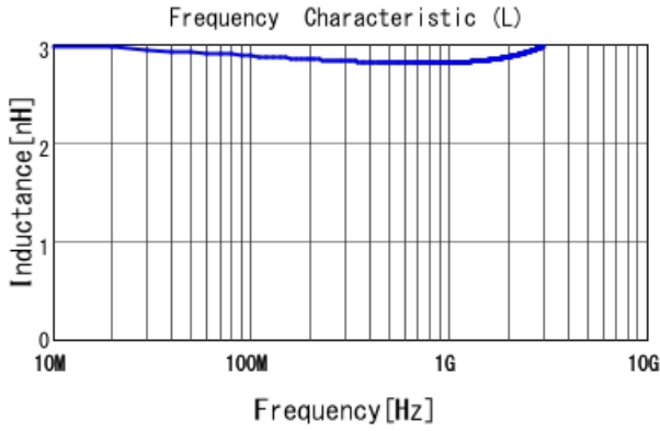
■ LQW15AN2N9B00 L
