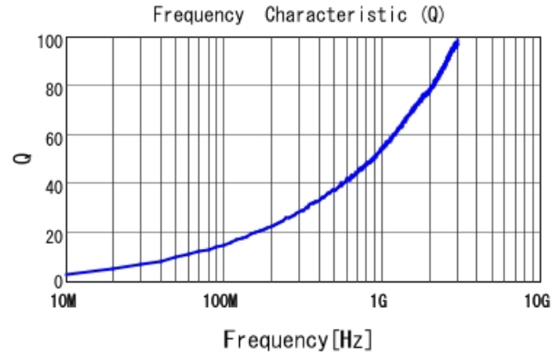
■ LQW15AN2N9B00 Q
