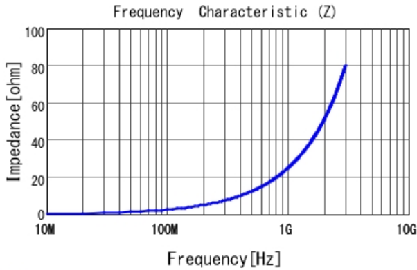
■ LQW15AN4N1B00 |Z|
