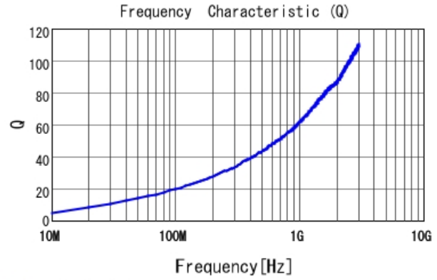
■ LQW15AN4N1B00 Q
