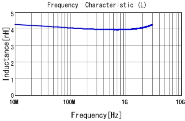
■ LQW15AN4N1B00 L
