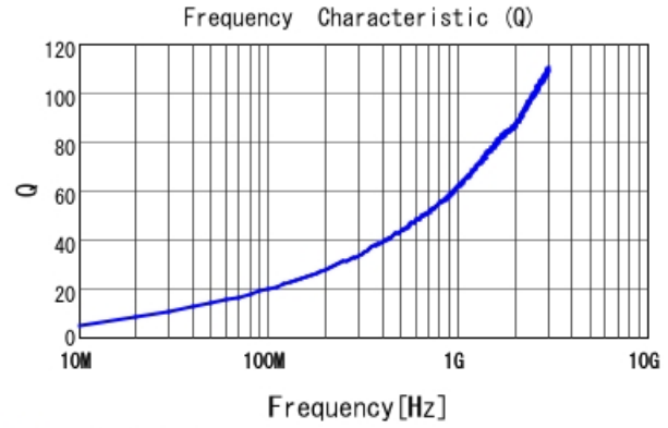
■ LQW15AN4N1C00 Q
