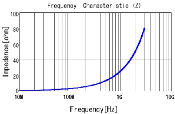
■ LQW15AN4N1C00 |Z|
