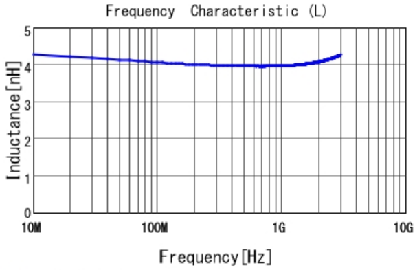
■ LQW15AN4N1C00 L
