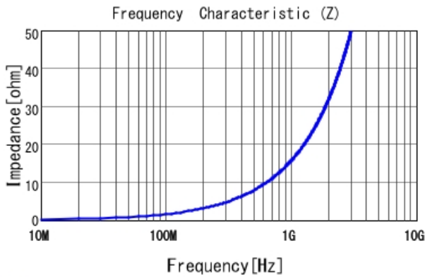
■ LQW15AN2N7C00 |Z|
