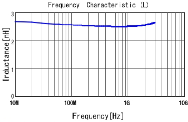
■ LQW15AN2N7C00 L
