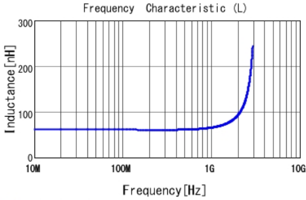
■ LQW15AN62NG00 L
