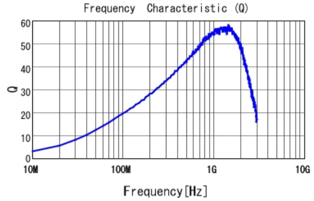
■ LQW15AN62NG00 Q
