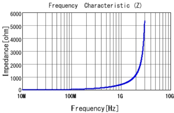
■ LQW15AN62NG00 |Z|
