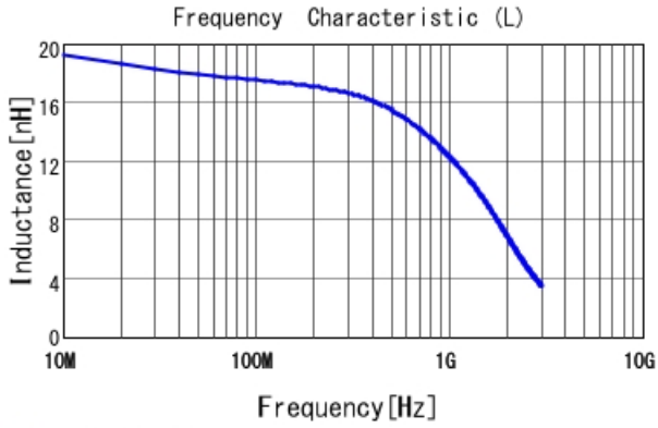
■ LQW15CN18NJ00 L
