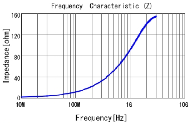
■ LQW15CN18NJ00 |Z|
