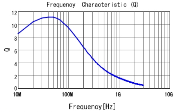
■ LQW15CN18NJ00 Q
