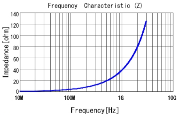
■ LQW15AN6N2B00 |Z|
