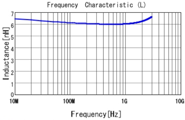
■ LQW15AN6N2B00 L
