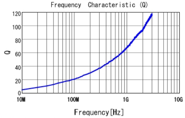
■ LQW15AN6N2B00 Q
