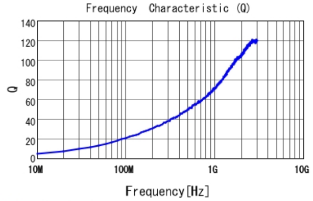
■ LQW15AN3N6C10 Q
