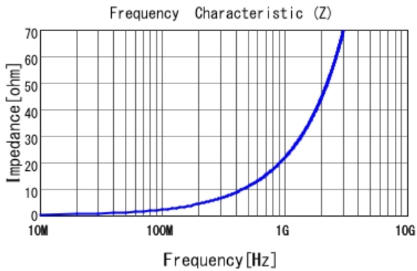
■ LQW15AN3N6C10 |Z|
