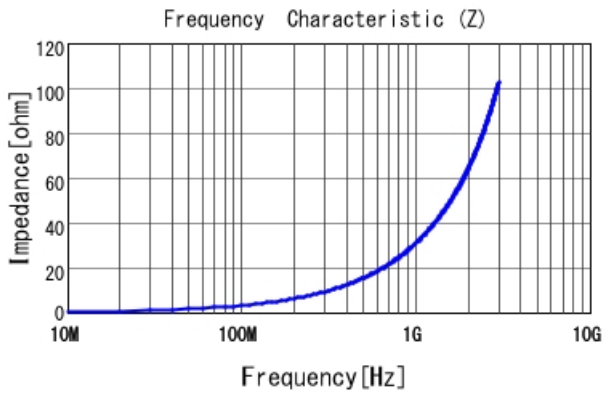
■ LQW15AN5N1B00 |Z|
