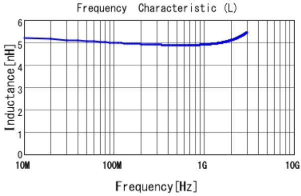
■ LQW15AN5N1B00 L
