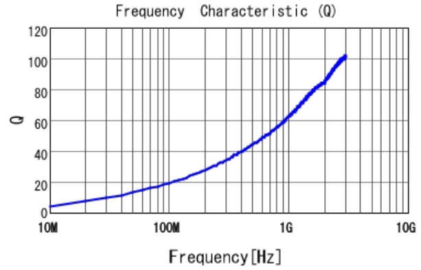
■ LQW15AN5N1B00 Q
