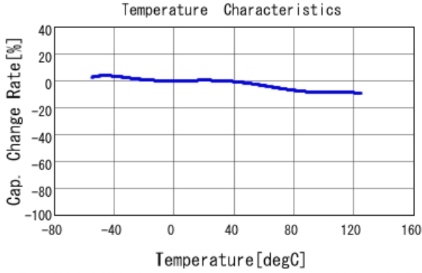
■ GCM155R71H102KA37 C-Temp. capchange, DCO. 0V, AC1. 0Vrm
