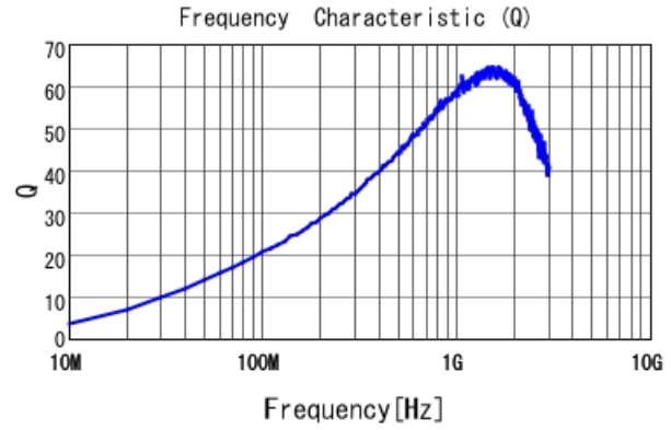
■ LQW15AN47NG00 Q
