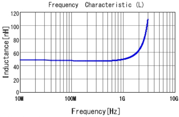
■ LQW15AN47NG00 L
