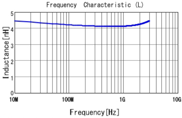
■ LQW15AN4N3B00 L
