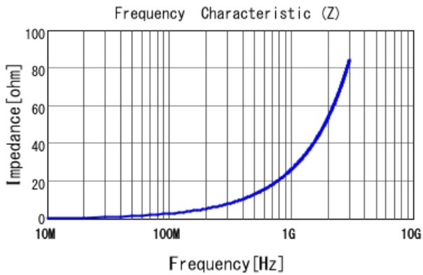
■ LQW15AN4N3B00 |Z|
