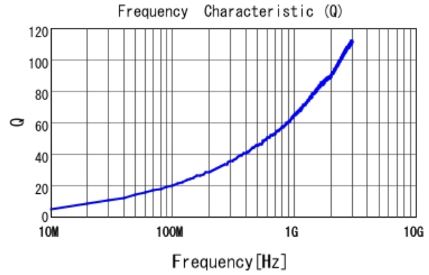
■ LQW15AN4N3B00 Q
