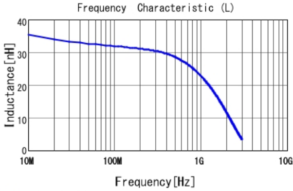
■ LQW15CN33NJ00 L
