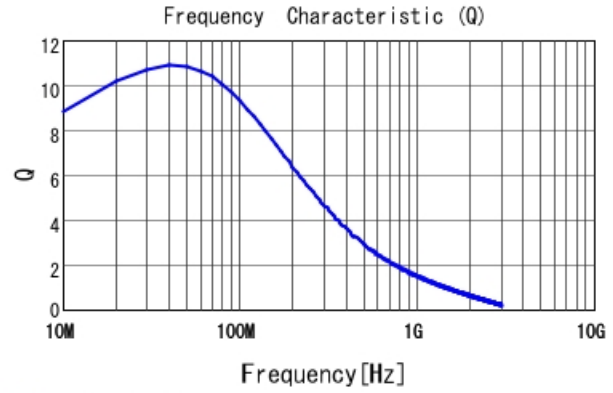
■ LQW15CN33NJ00 Q
