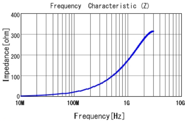
■ LQW15CN33NJ00 |Z|
