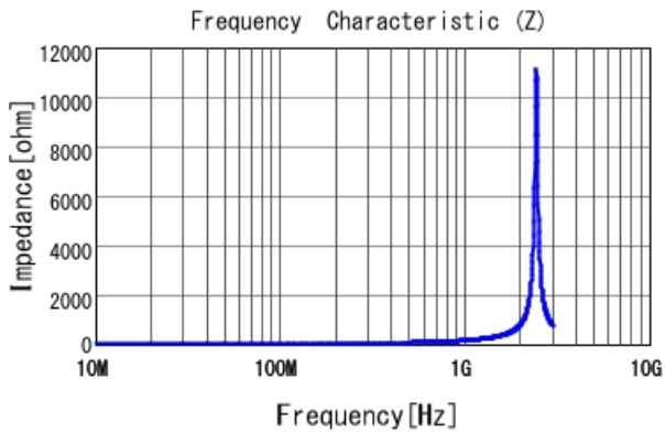
■ LQG15HN22NJ02 |Z|
