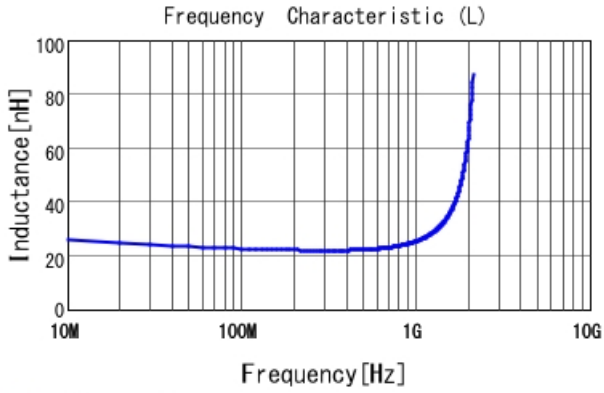
■ LQG15HN22NJ02 L
