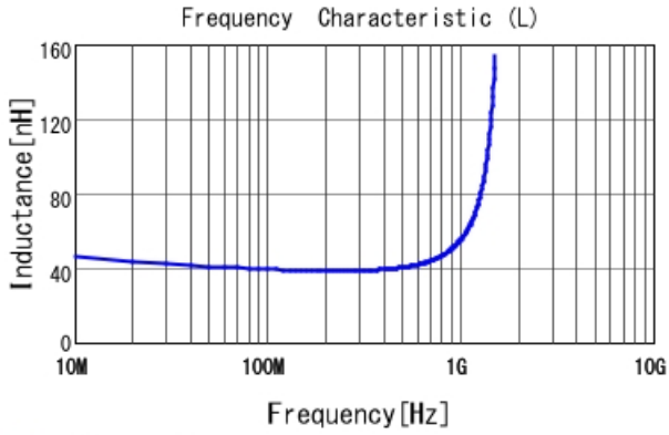
■ LQG15HN39NJ02 L
