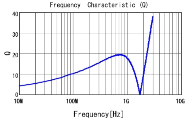
■ LQG15HN39NJ02 Q
