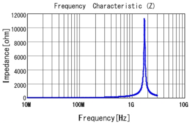
■ LQG15HN39NJ02 |Z|
