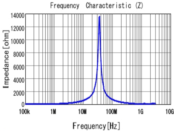
■ LQH5BPH100MT0 |Z|
