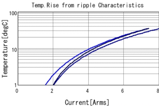
GRM32EC70J107ME15 Temp. rise ■ 50kHz ■ 200kHz ■ 400kHz
